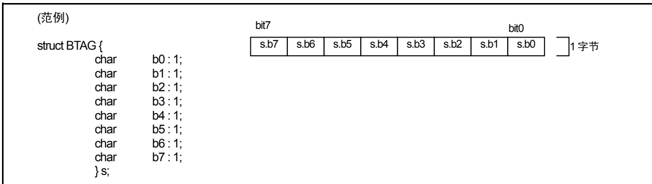
图 D.7 位字段的布局范例 (1)
