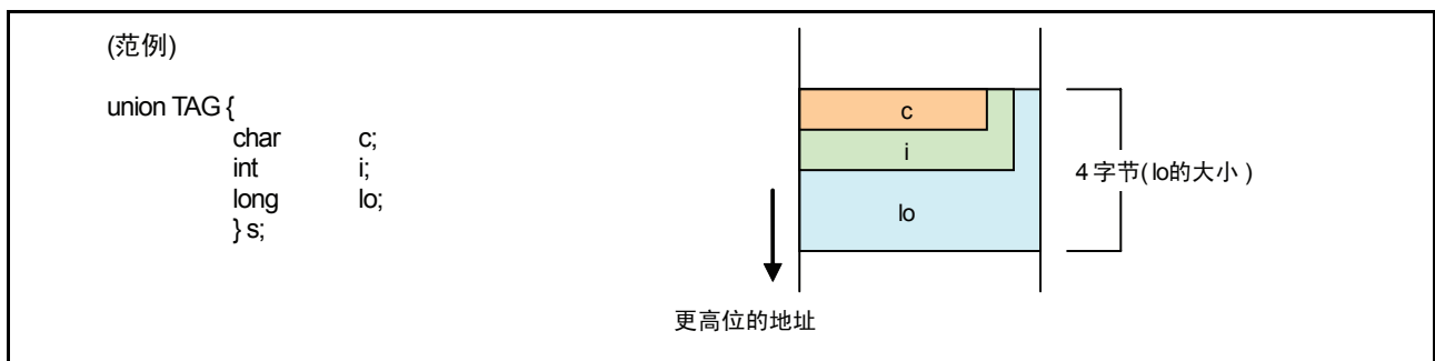
图 D.6 联合的布局范例
