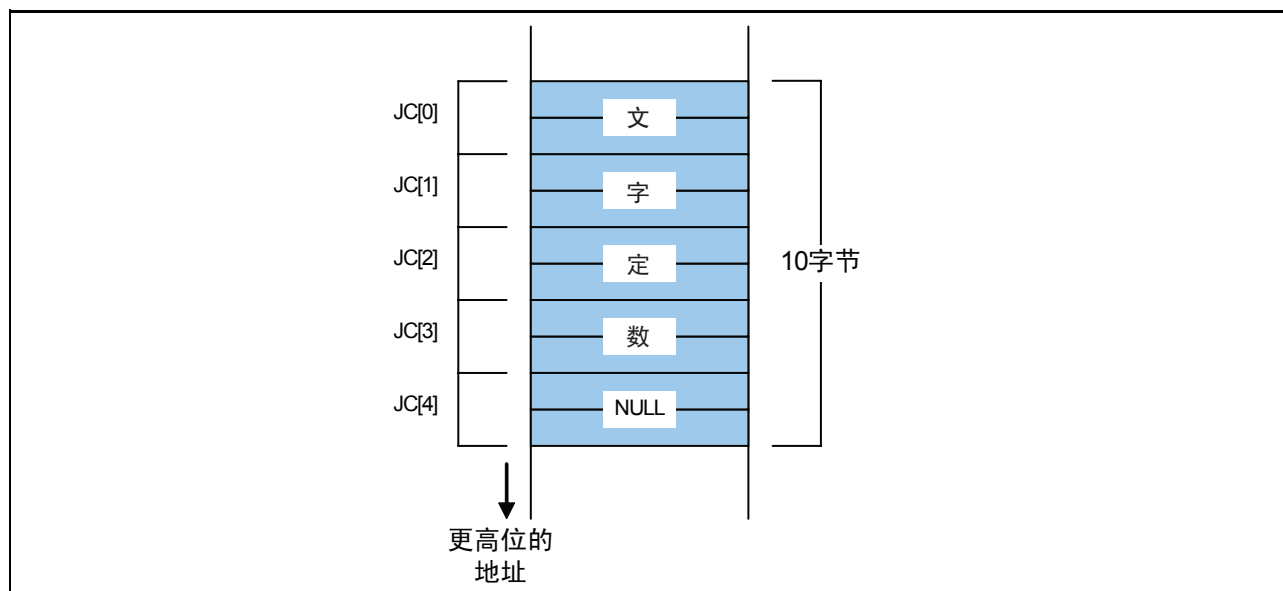
图 B.46 wchar_t 类型字符常数所分配数组的存储器位置
