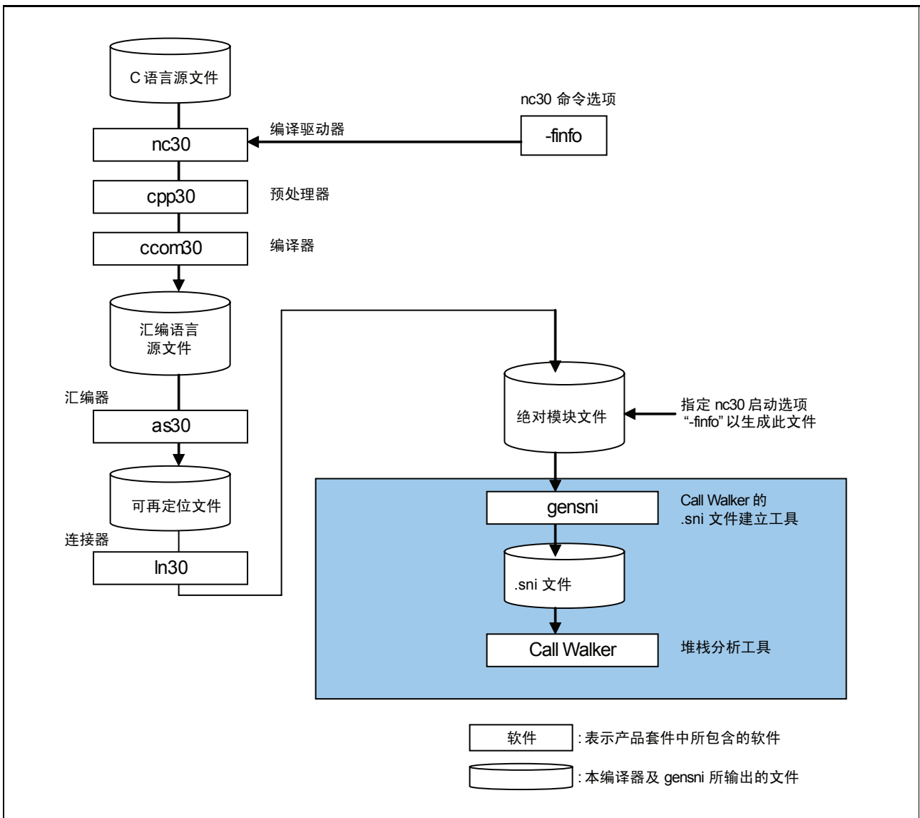
图 H.1 NC30 的处理流程
