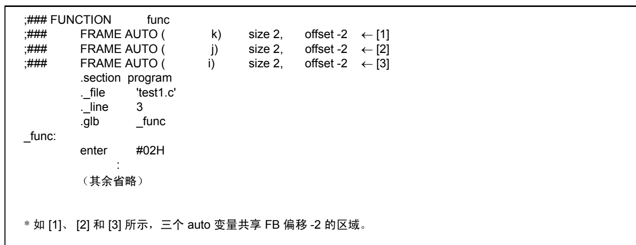
图 D.21 汇编语言源程序的范例
