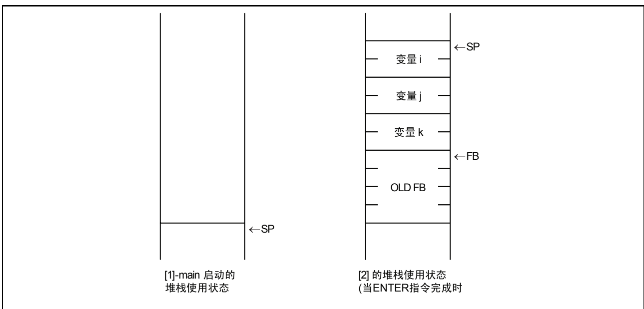
图 D.17 函数 main 的进入处理
