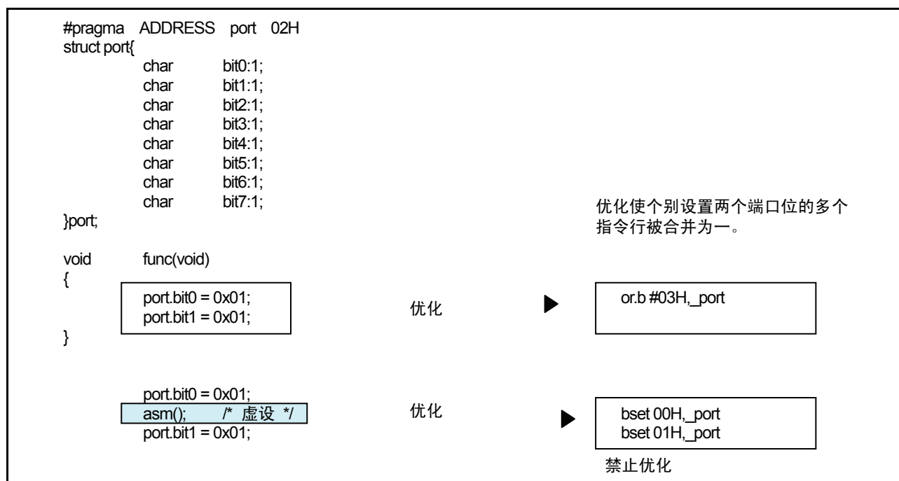
图 B.34 使用虚设 asm 来禁止优化的范例
