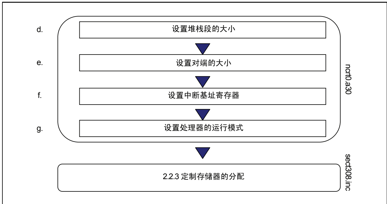
图 2.11 修改启动程序的范例步骤
