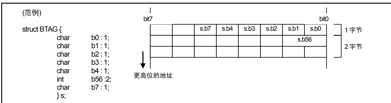
图 D.8 位字段的布局范例 (2)
