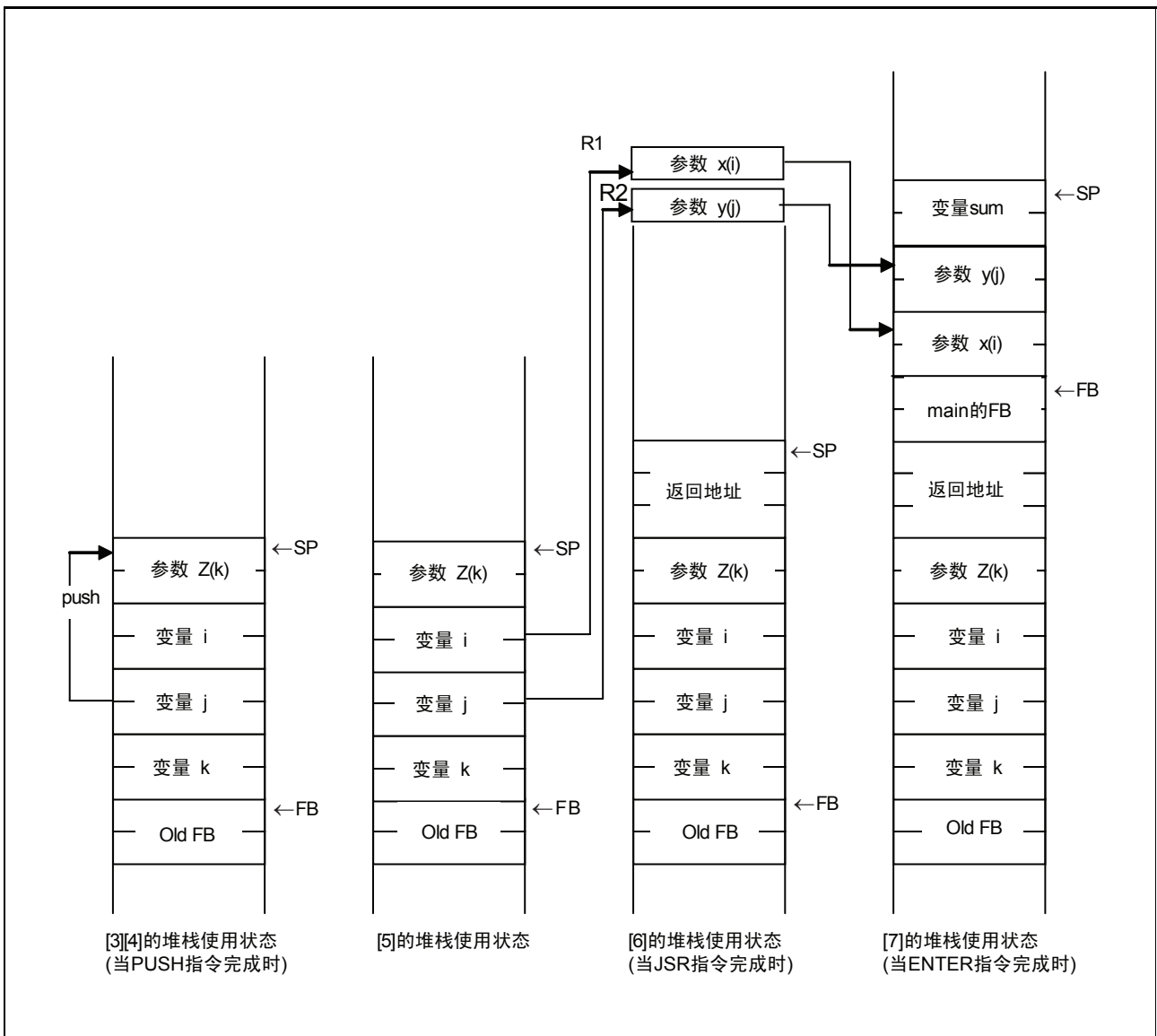
图 D.18 调用函数 func 和进入处理
