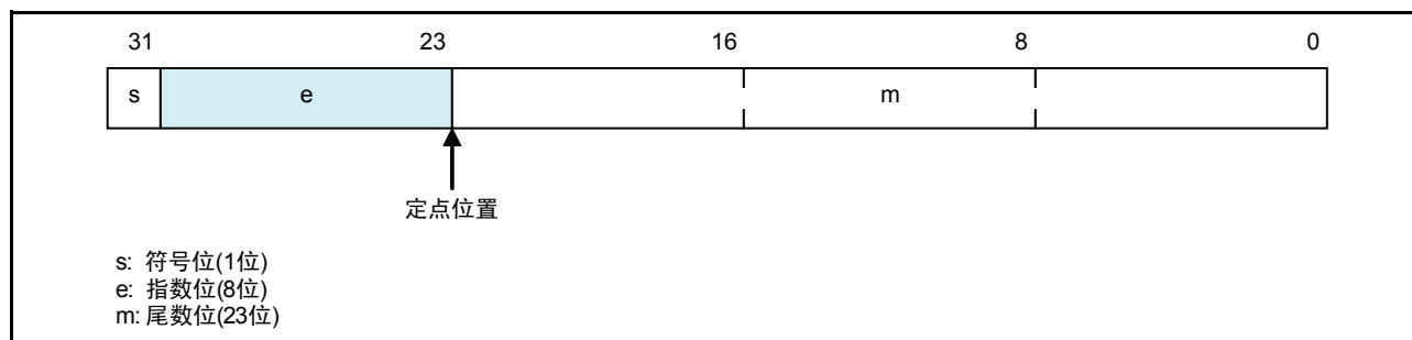
图 D.1 单精度浮点数据格式
