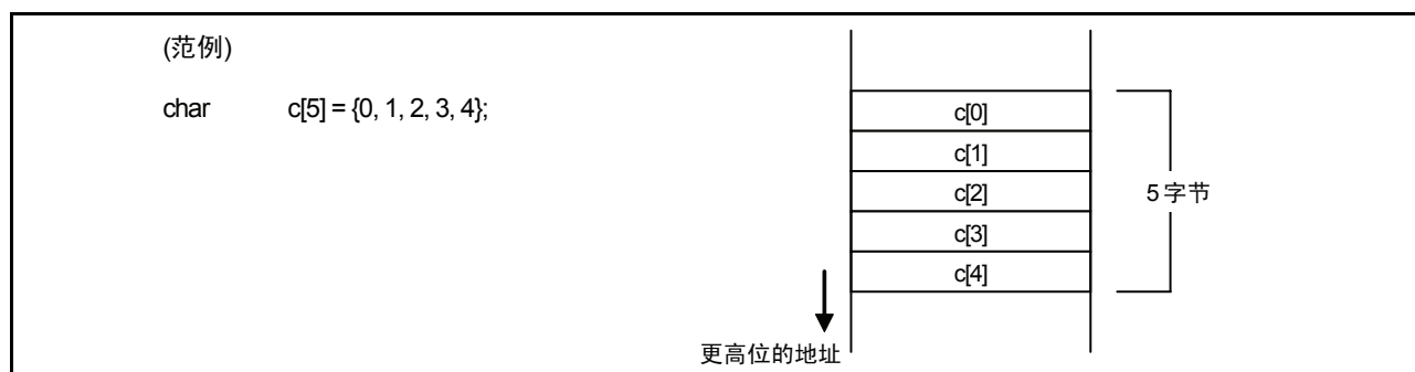
图 D.3 数组的布局范例
