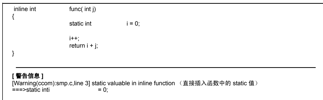
图 B.59 直接插入函数的错误编码范例 (4)
