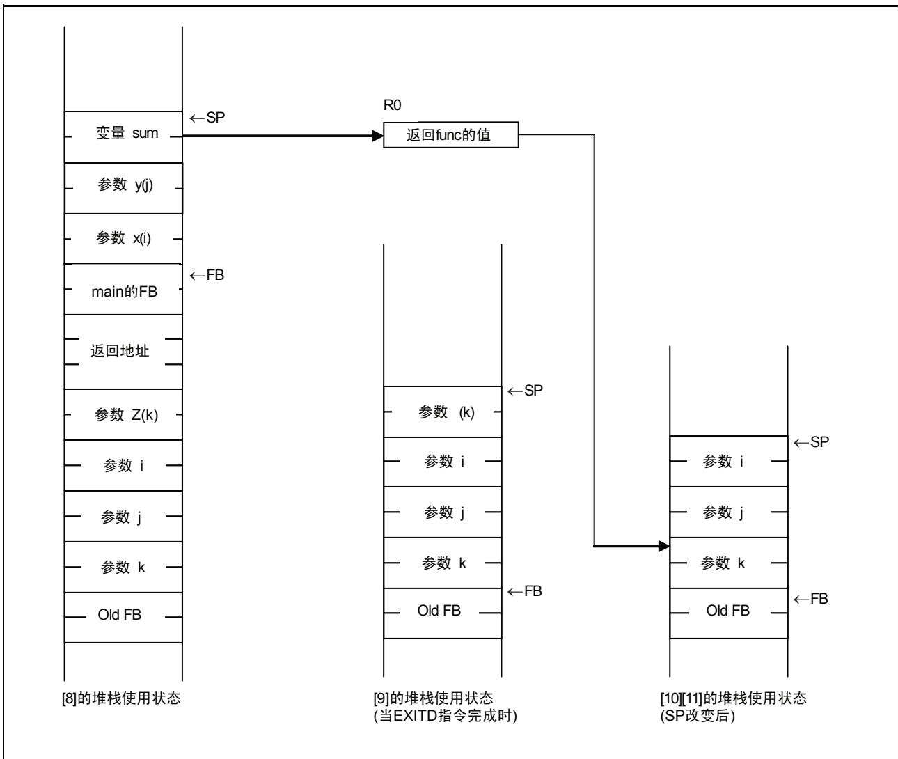
图 D.19 函数 func 的退出处理
