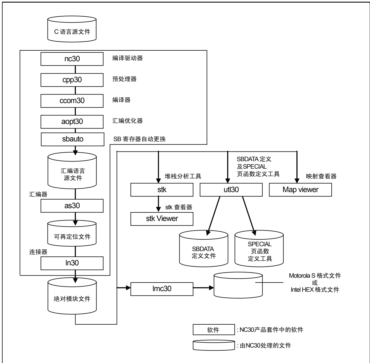
图 1.1 NC30 处理流程
