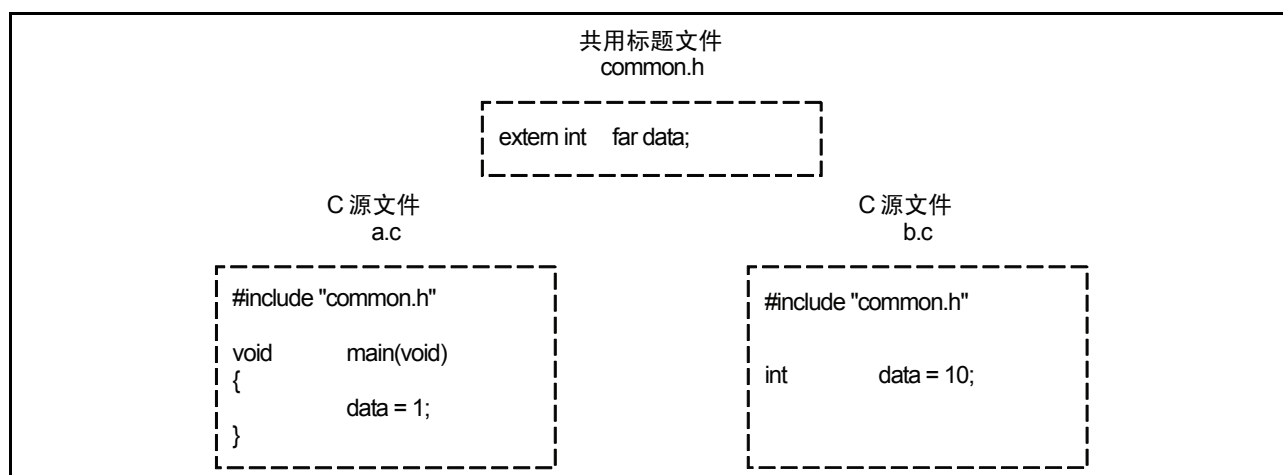
图 B.14 共用标题文件声明的范例
