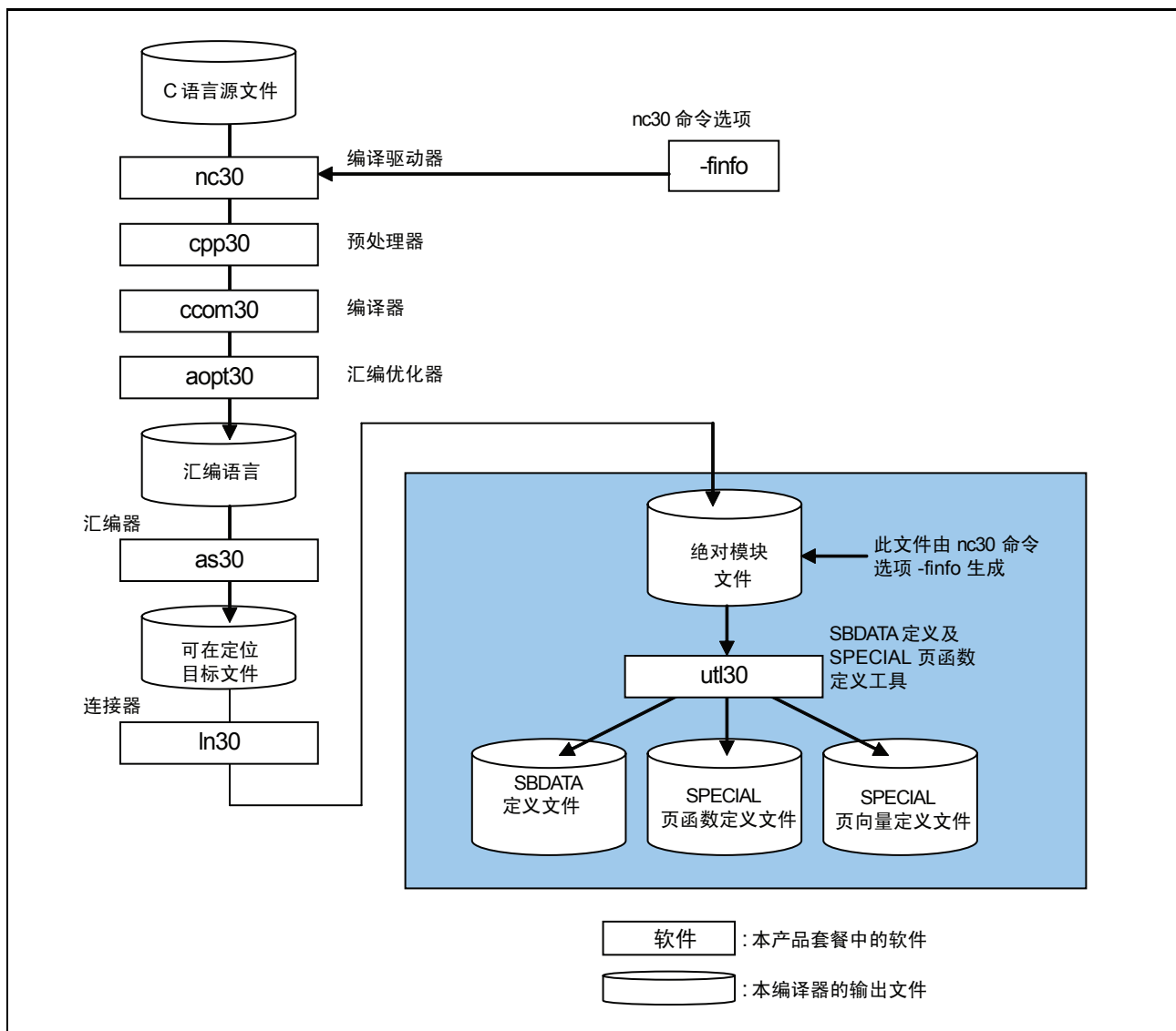
图 G.1 NC30 处理流程
