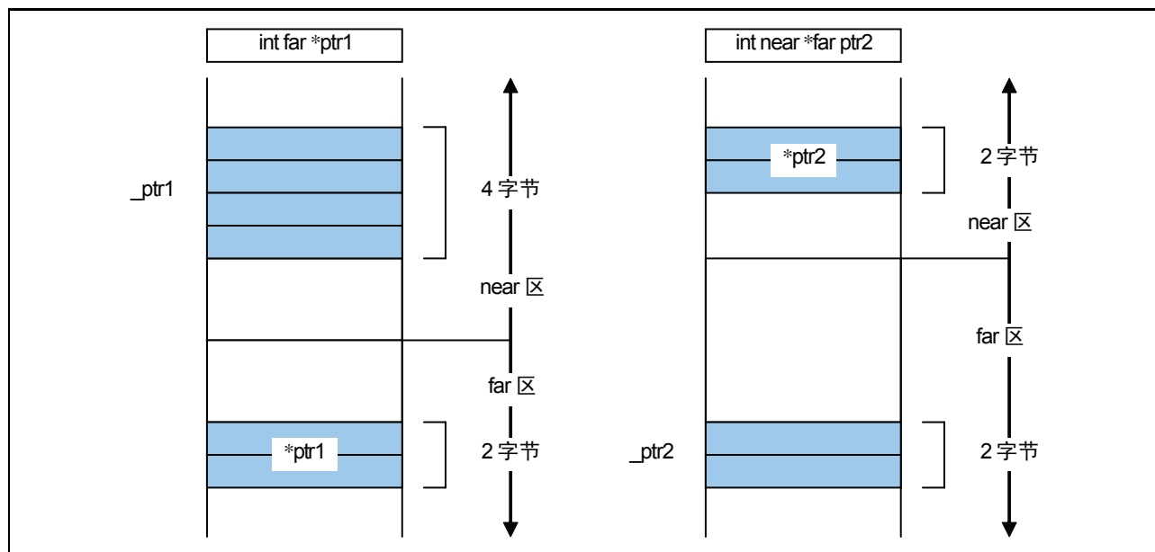
图 B.9 指针类型变量的存储器位置
