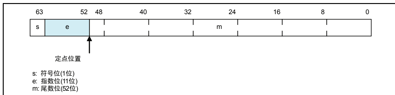
图 D.2 双精度浮点数据格式
