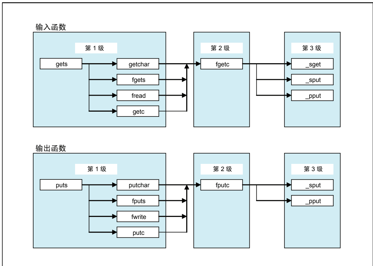
图 E.1 I/O 函数的调用关系
