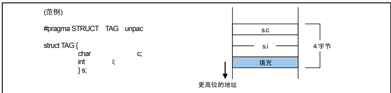
图 D.5 结构的布局范例 (2)
