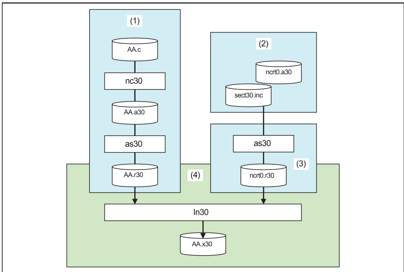
图 1.3 程序开发流程
