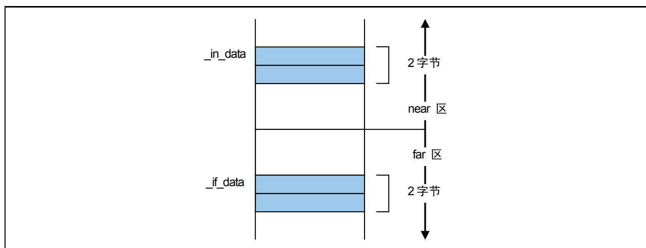
图 B.3 变量的存储器位置
