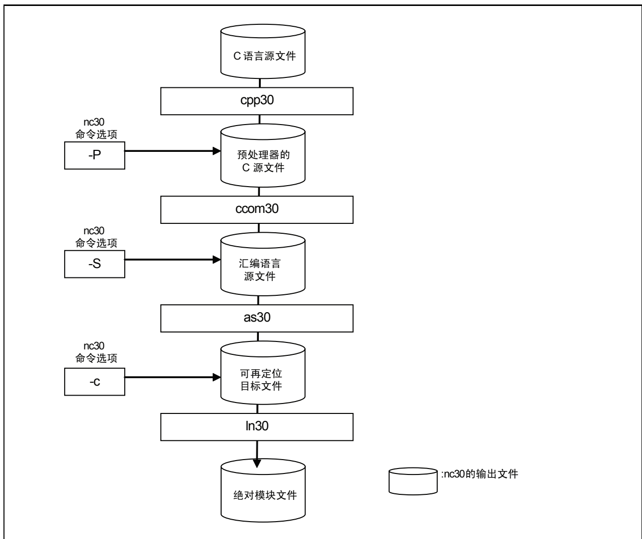
图 1.6 NC30 命令行选项与输出文件的关系
