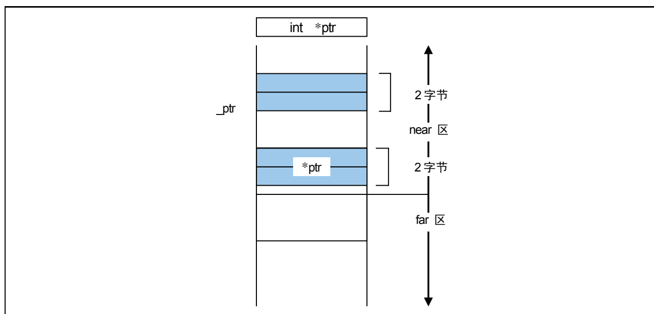
图 B.6 指针类型变量的存储器位置
